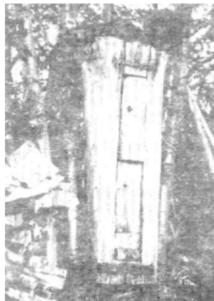
Колодный улей.
